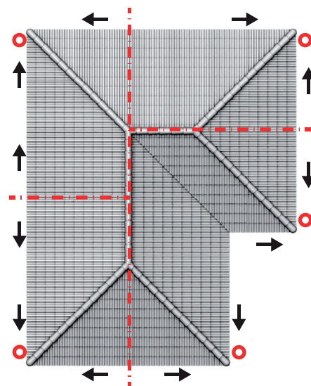
Кровля с несколькими стоками
